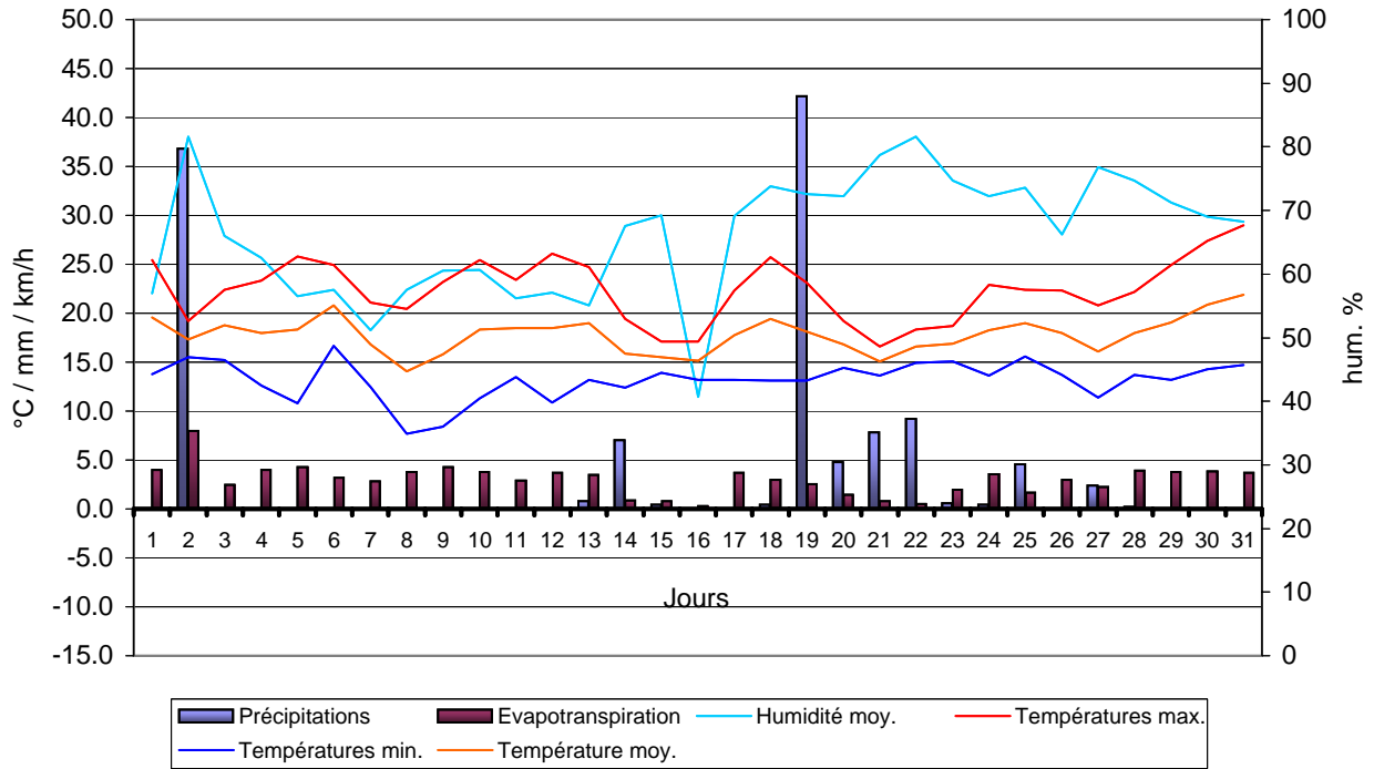
Précipitations - Etp. - Température - Humidité - Vents - Août 2005 Valeyres-sous-Montagny - www.meteo-vsm.ch
