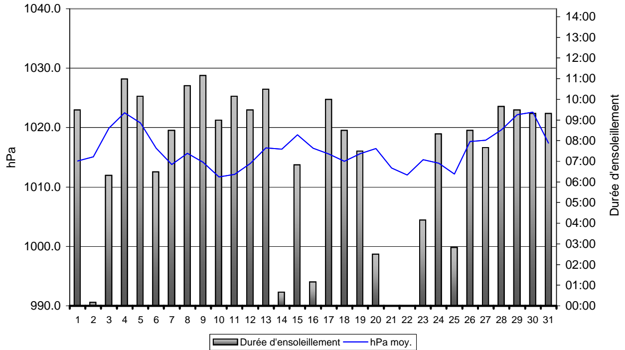
Pressions atm. moyennes - Durée d'ensoleillement - Août 2005 Valeyres-sous-Montagny - www.meteo-vsm.ch
