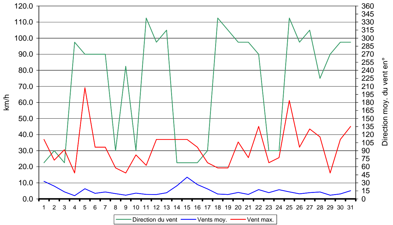
Direction du vent - Vitesse max. - Vitesse moy. - Juillet 2006 Valeyres-sous-Montagny - www.meteo-vsm.ch
