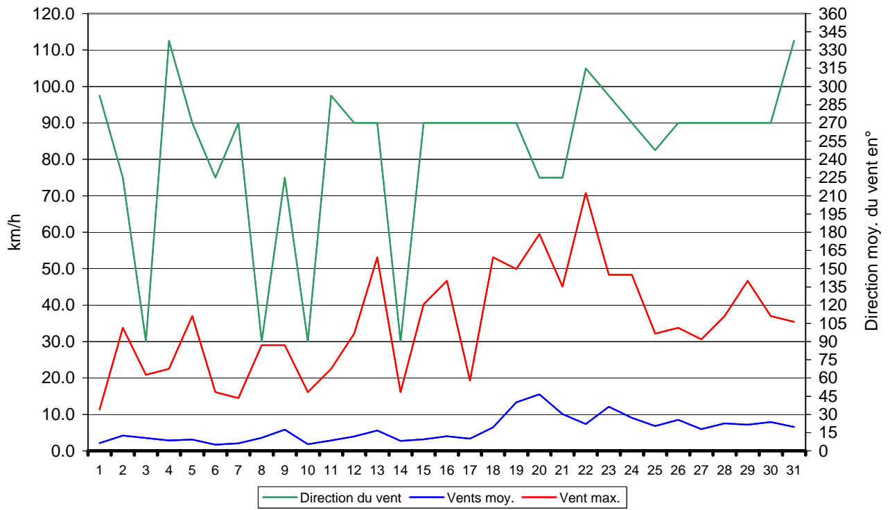
Direction du vent - Vitesse max. - Vitesse moy. - Mai 2006 Valeyres-sous-Montagny - www.meteo-vsm.ch
