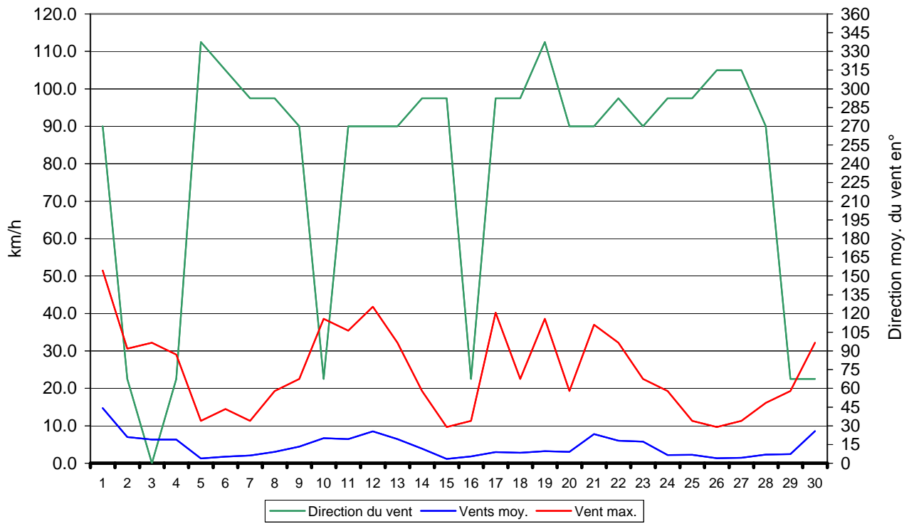
Direction du vent - Vitesse max. - Vitesse moy. - Novembre 2006 Valeyres-sous-Montagny - www.meteo-vsm.ch
