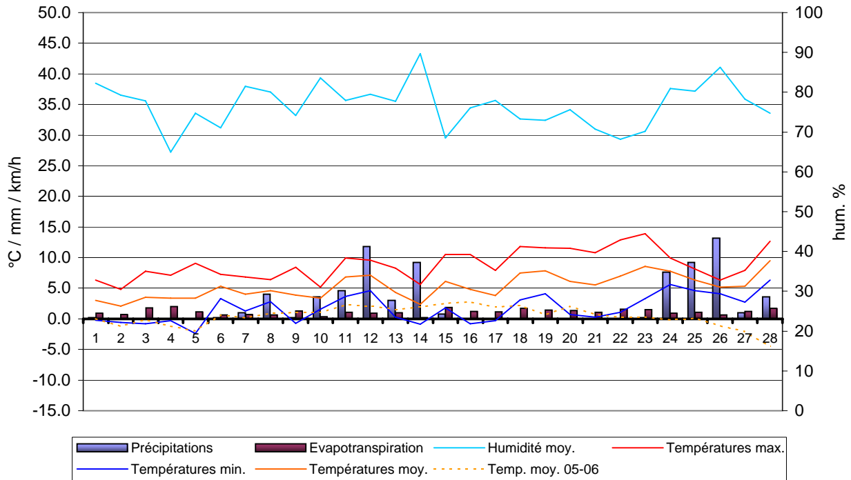
Précipitations - Etp. - Température - Humidité - Vents - Février 2007 Valeyres-sous-Montagny - www.meteo-vsm.ch
