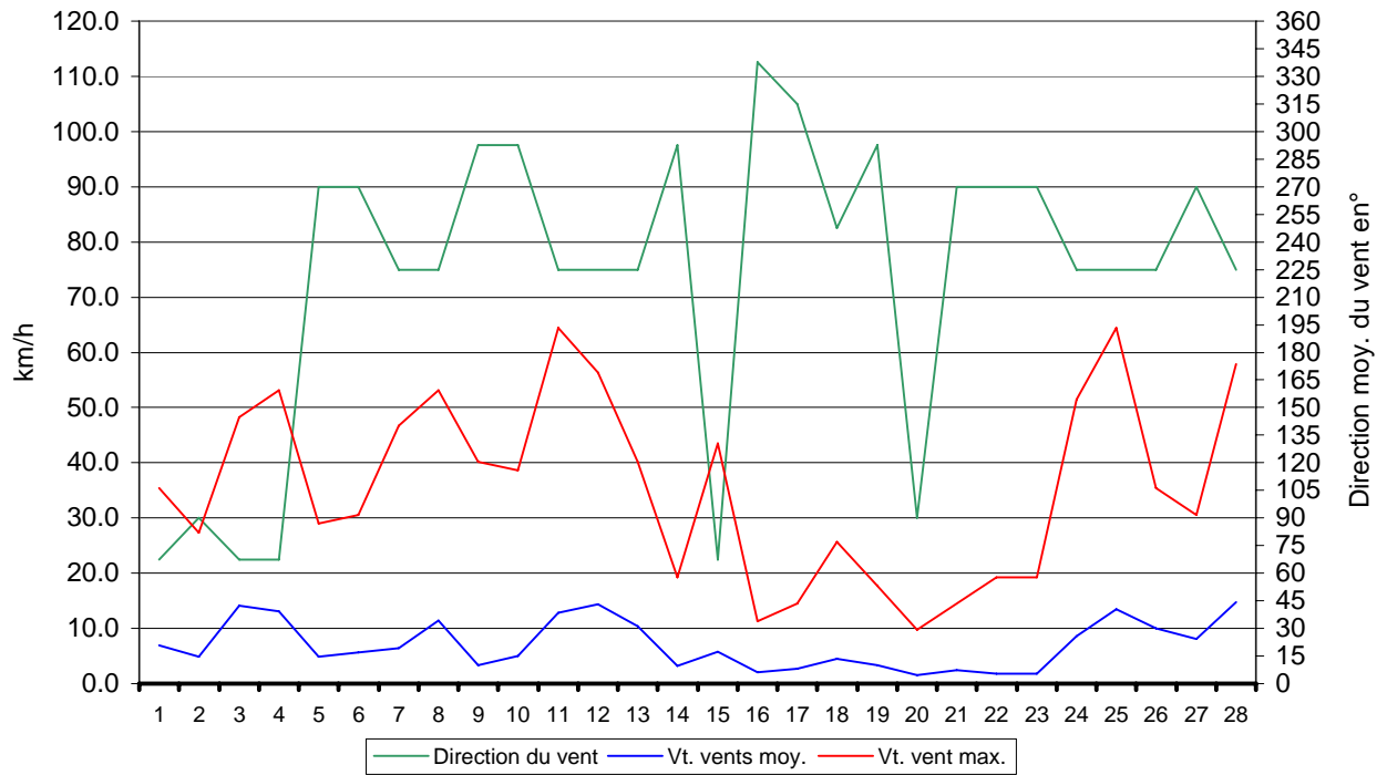
Direction du vent - Vitesse max. - Vitesse moy. - Février 2007 Valeyres-sous-Montagny - www.meteo-vsm.ch
