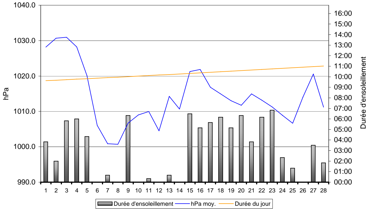
Pressions atm. moyennes - Durée d'ensoleillement - Février 2007 Valeyres-sous-Montagny - www.meteo-vsm.ch
