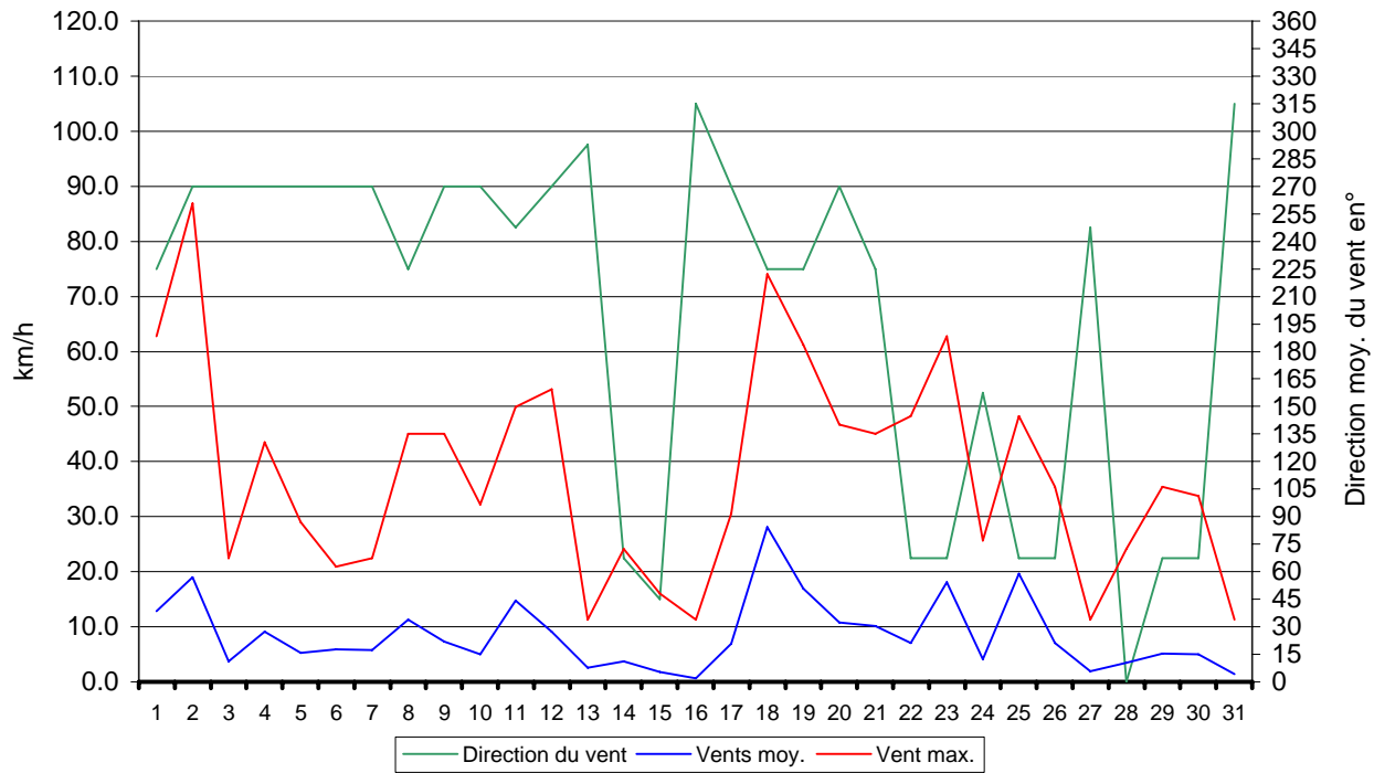
Direction du vent - Vitesse max. - Vitesse moy. - Janvier 2007 Valeyres-sous-Montagny - www.meteo-vsm.ch
