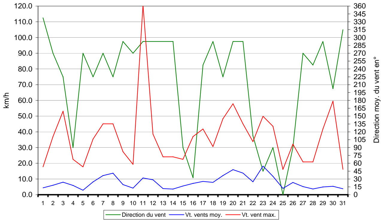
Direction du vent - Vitesse max. - Vitesse moy. - Juillet 2008 Valeyres-sous-Montagny - www.meteo-vsm.ch
