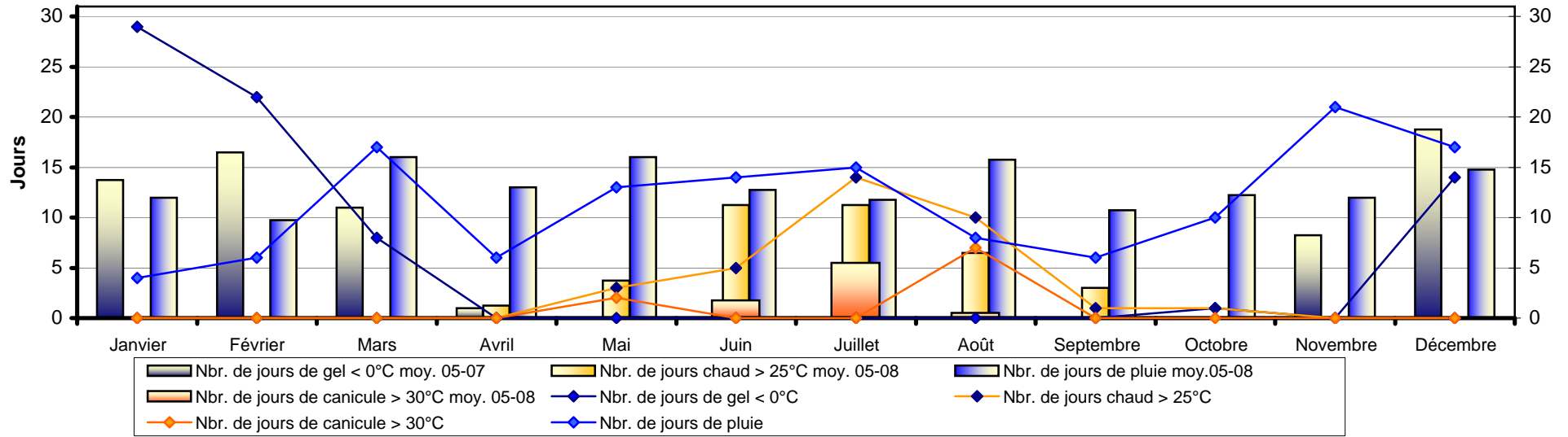
Nbr de jours de gel < 0°C, de chaud > 25°C, de canicule >30°C, de pluie Valeyres-sous-Montagny 2009 - www.meteo-vsm.ch
