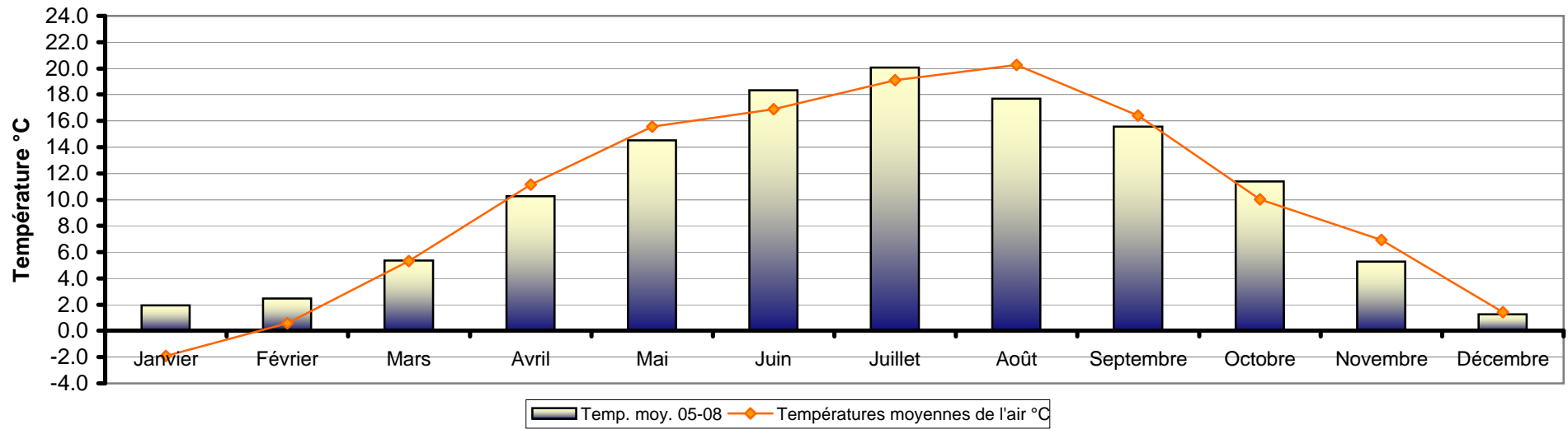
Températures moy. de l'air à +200cm en °C Valeyres-sous-Montagny 2009 - www.meteo-vsm.ch
