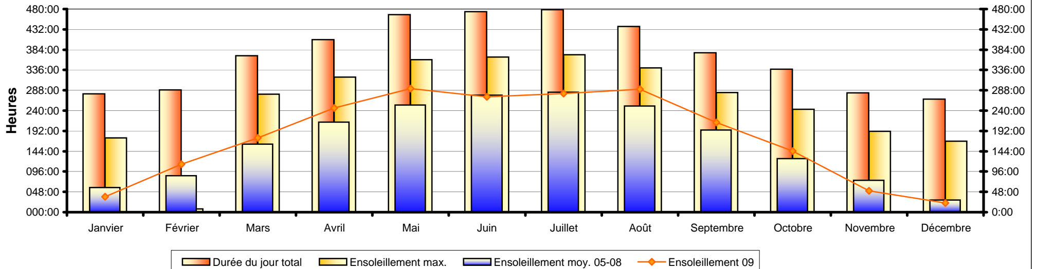
Ensoleillement Valeyres-sous-Montagny 2009 - www.meteo-vsm.ch
