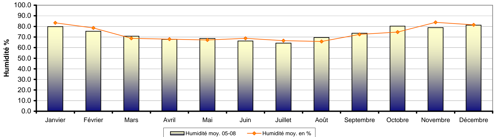
Humidité moy. de l'air à +200cm en % Valeyres-sous-Montagny 2009 - www.meteo-vsm.ch
