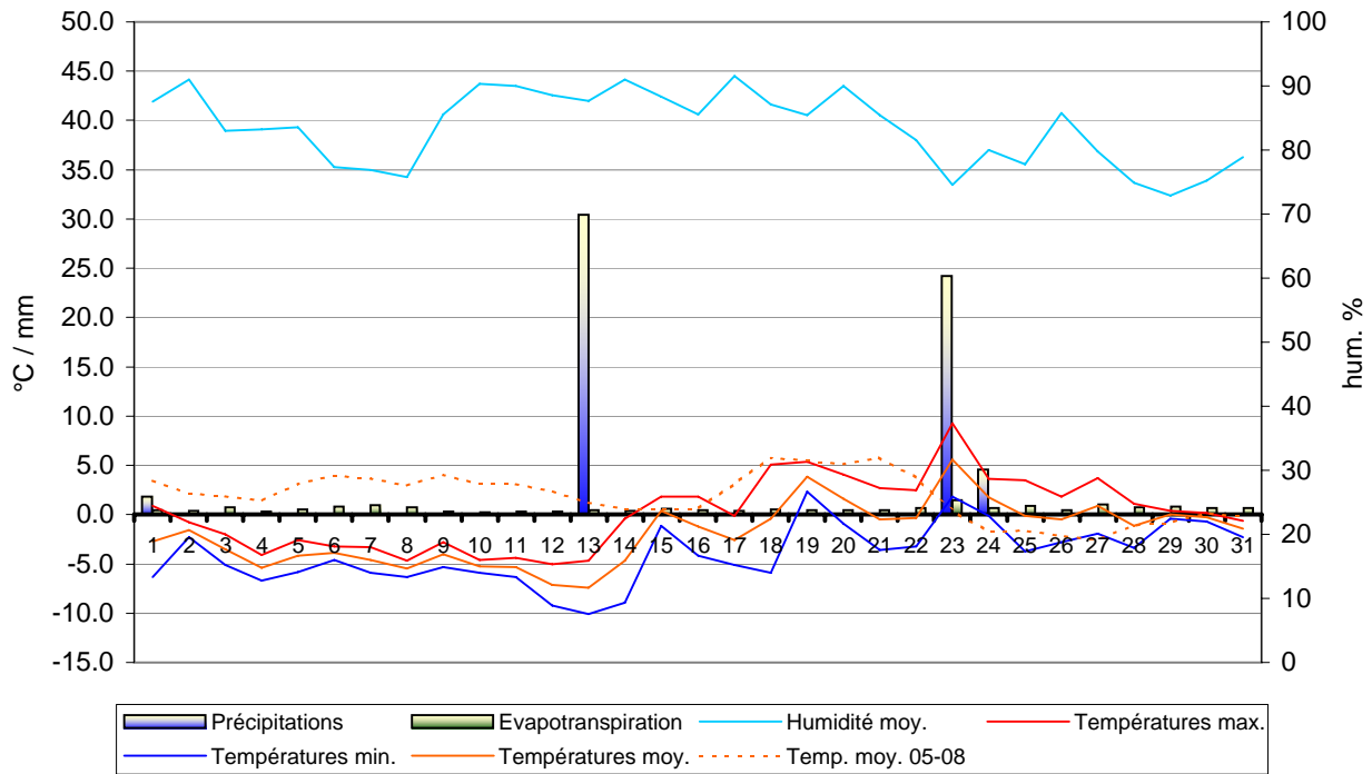
Précipitations - Etp. - Température - Humidité - Vents - Janvier 2009 Valeyres-sous-Montagny - www.meteo-vsm.ch
