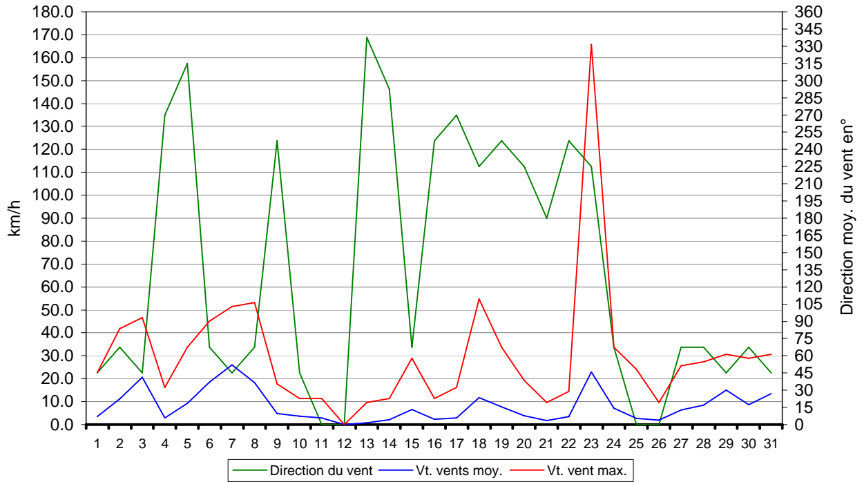
Direction du vent - Vitesse max. - Vitesse moy. - Janvier 2009 Valeyres-sous-Montagny - www.meteo-vsm.ch
