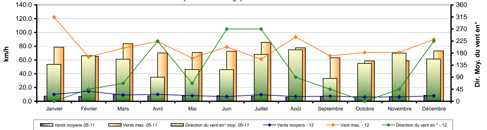
Direction moy. du vent - Vitesse max. - Vitesse moy. Valeyres-sous-Montagny 2012 - www.meteo-vsm.ch
