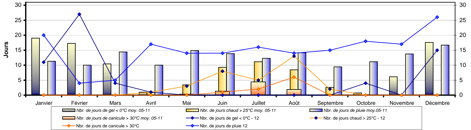
Nbr de jours de gel < 0°C, de chaud > 25°C, de canicule >30°C, de pluie Valeyres-sous-Montagny 2012 - www.meteo-vsm.ch
