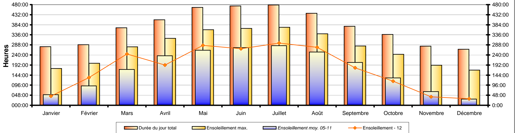
Ensoleillement Valeyres-sous-Montagny 2012 - www.meteo-vsm.ch
