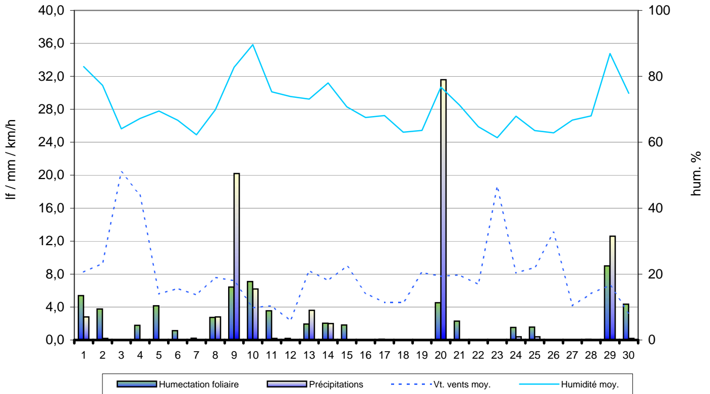
Température de l'air, du sol - Humidité du sol - Juin 2013 Valeyres-sous-Montagny - www.meteo-vsm.ch
