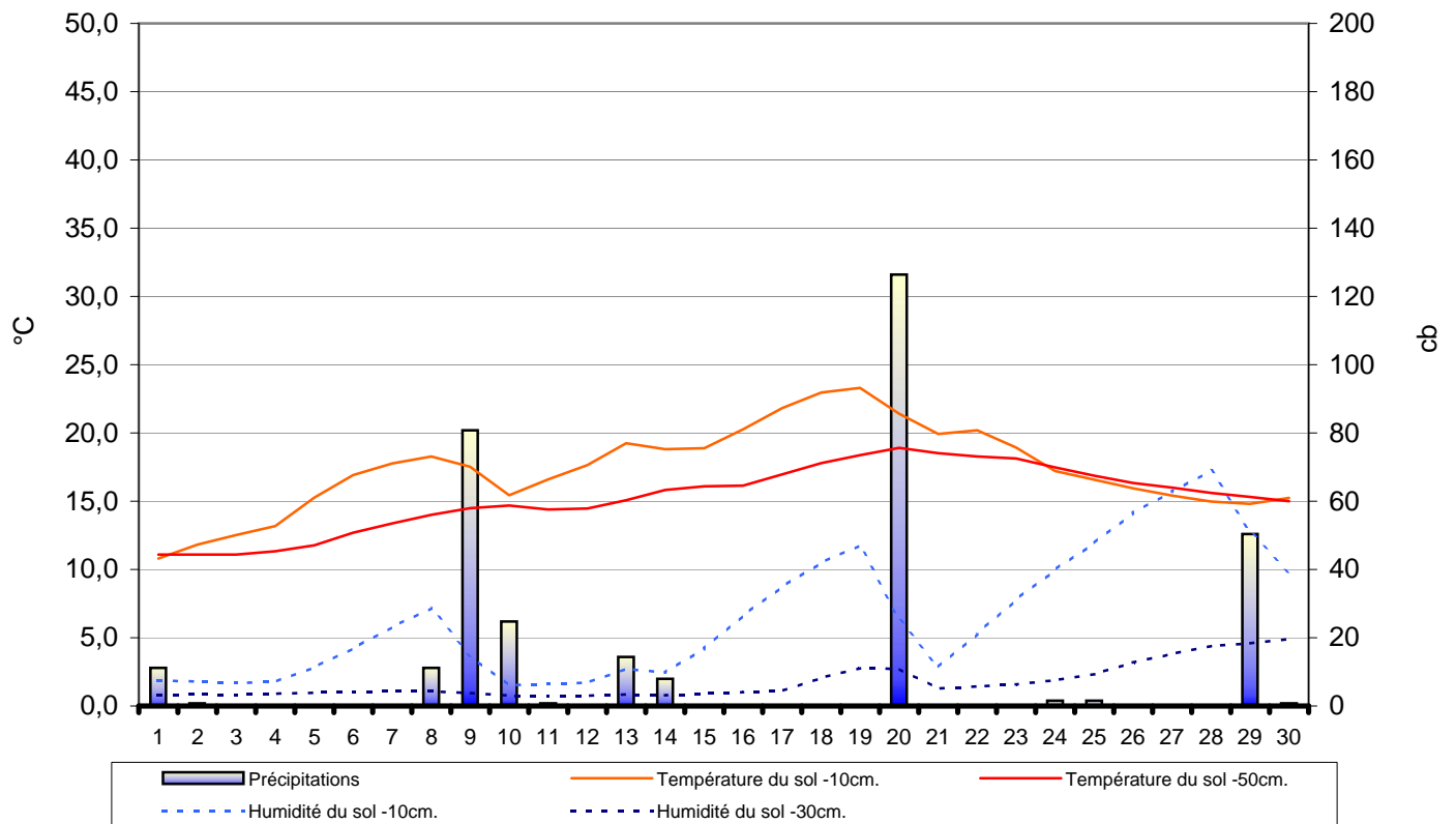
Température de l'air, du sol - Humidité du sol - Juin 2013 Valeyres-sous-Montagny - www.meteo-vsm.ch
