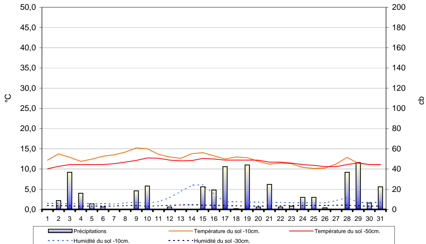
Température de l'air, du sol - Humidité du sol - Mai 2013 Valeyres-sous-Montagny - www.meteo-vsm.ch
